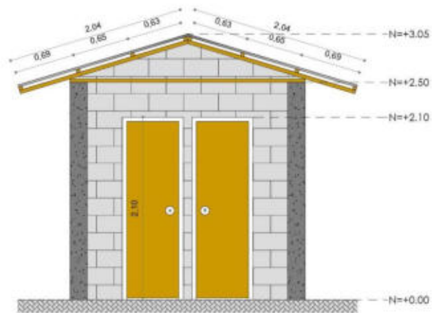
ELEVACIÓN FRONTAL
