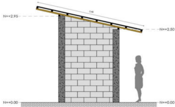
ELEVACIÓN LATERAL IZQUIERDA escala 1:50
