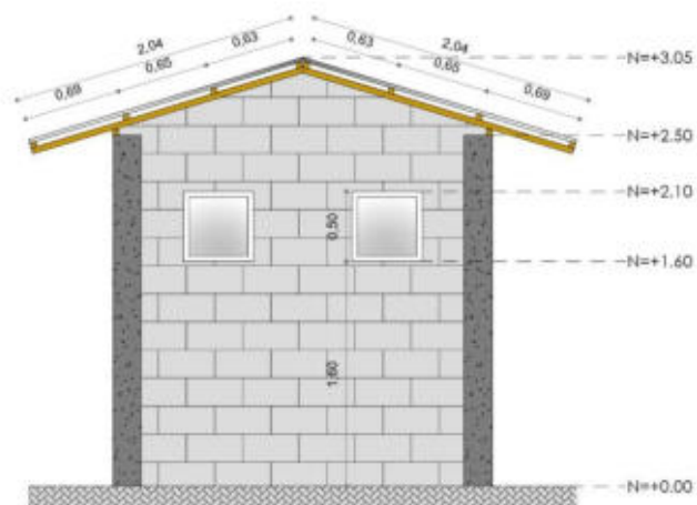
ELEVACIÓN POSTERIOR
