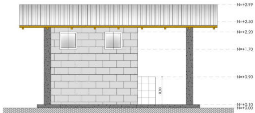
ELEVACIÓN POSTERIOR
